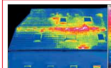
Problema isolamento tetto
