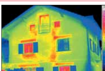
Perdite di calore
