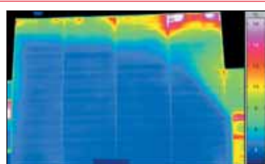
Fughe termiche (edificio industriale)
