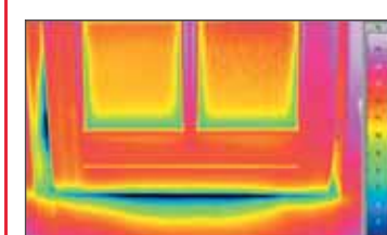
Individuazione problemi di isolamento (con metodo Blower Door)
