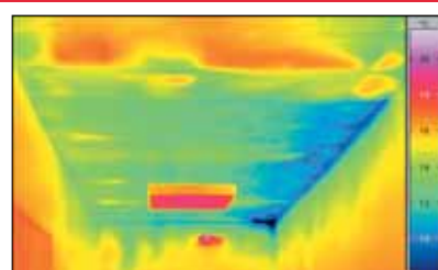
Isolamento soffitto
