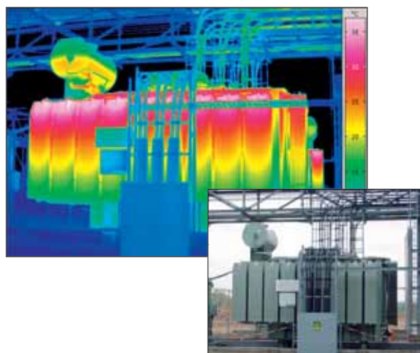
Ispezione di trasformatori
