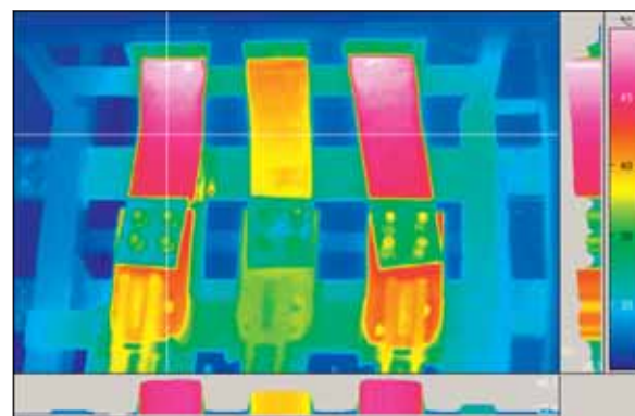
Riscaldamento conduttori con differente carica
