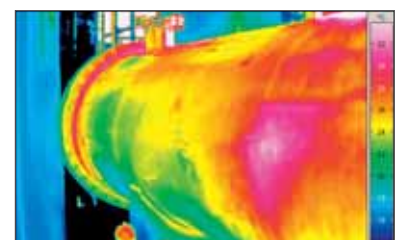
Difetto di isolamento
