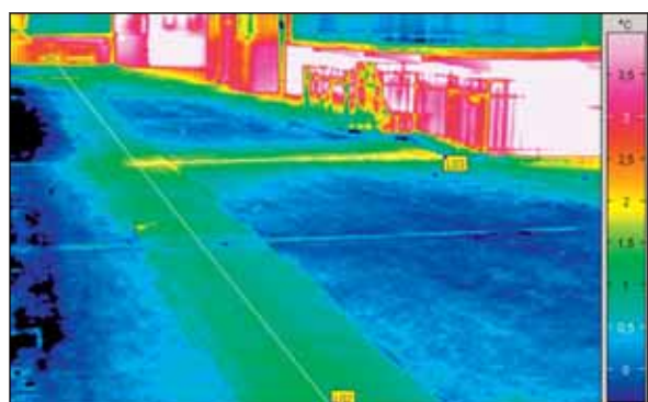
Tubi di riscaldamento sotterranei
