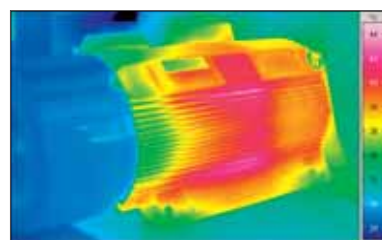
Controllo temperatura motori
