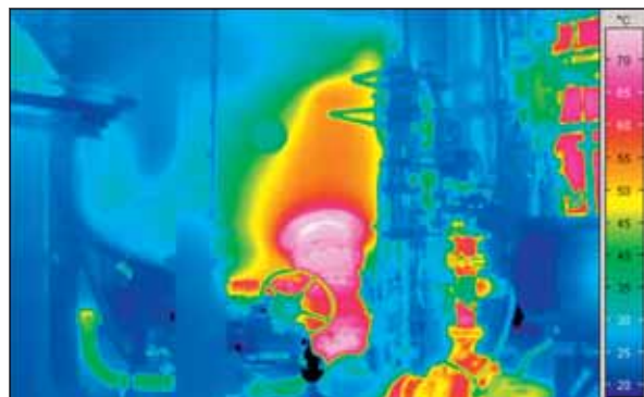
Uscita prodotti da reattore
